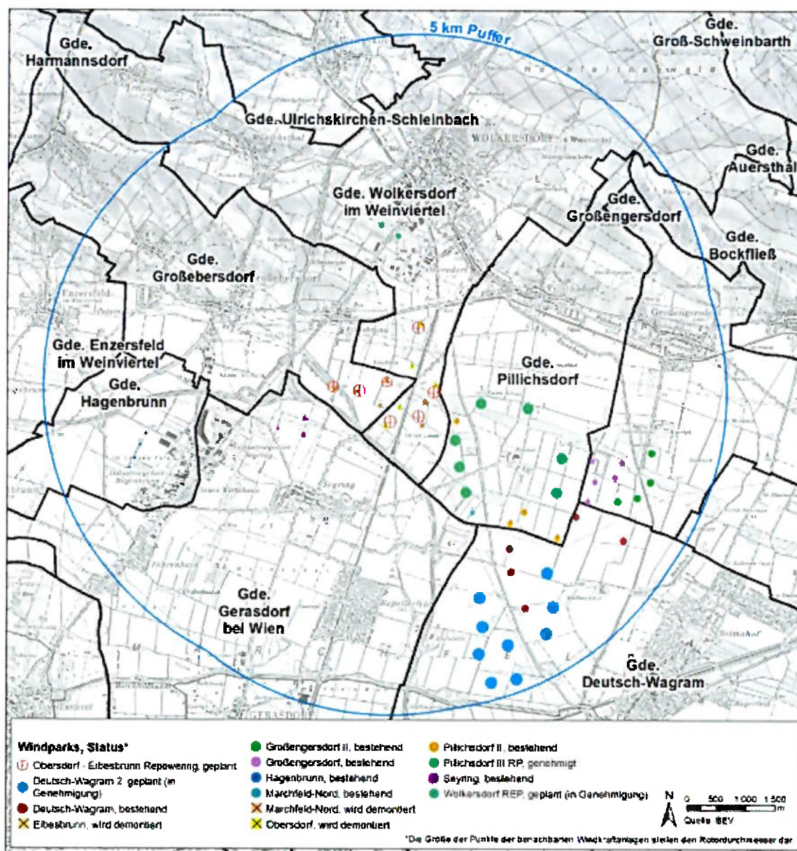
Abbildung: Übersichtsplan Windpark Obersdorf – Eibesbrunn Repowering
