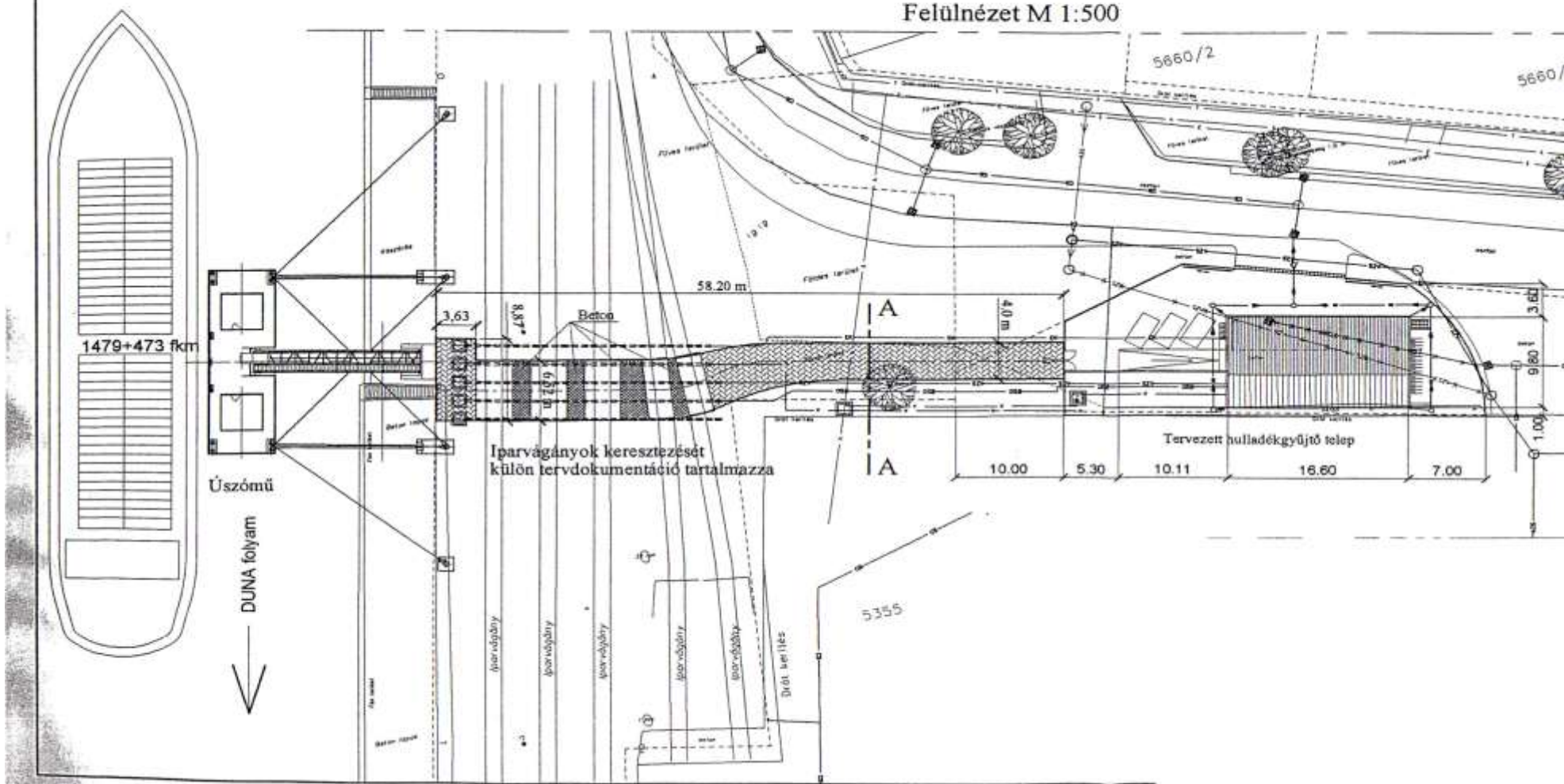
Felülnézet M 1:500
